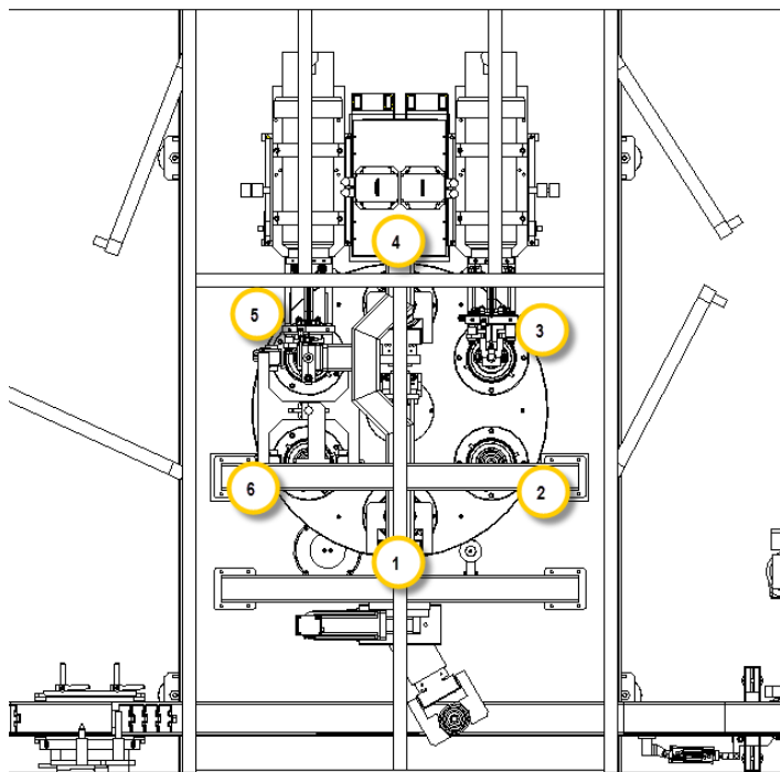
Fig.6 indexing table diagram.
